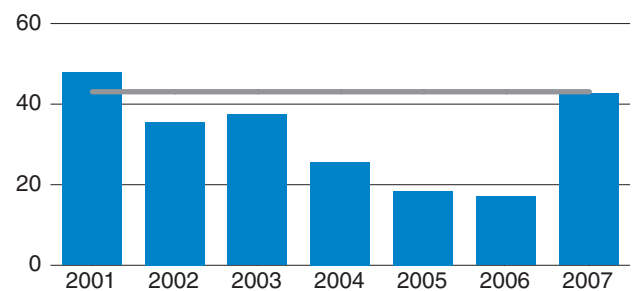
BOD utsläpp från avloppsreningsverken 2001-2007 (ton/år)
