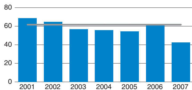
Kväveutsläpp från avloppsreningsverken 2001-2007 (ton/år)
