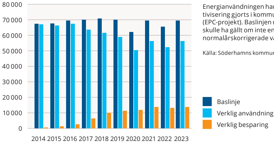
Energianvändning i fastigheter som ingår i EPC-projekt (MWh per år)
